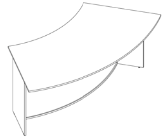
60° Outer Curved DDA VRCCD60*-** 2100(w) x 900(d) x 760(h)mm
