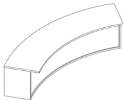
60° Inner Curved Mid VRTCM61* -** 1700(w) x 400(d) x 400(h)mm
